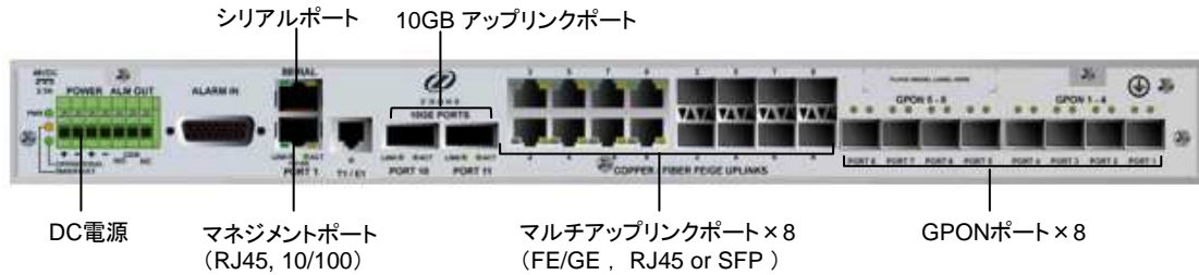
<XP-198-10GE 前面>
